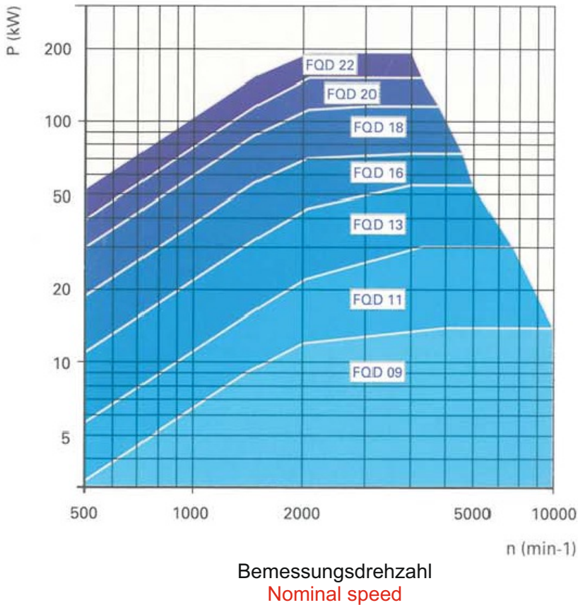
Leistungsübersicht Power rating chart
