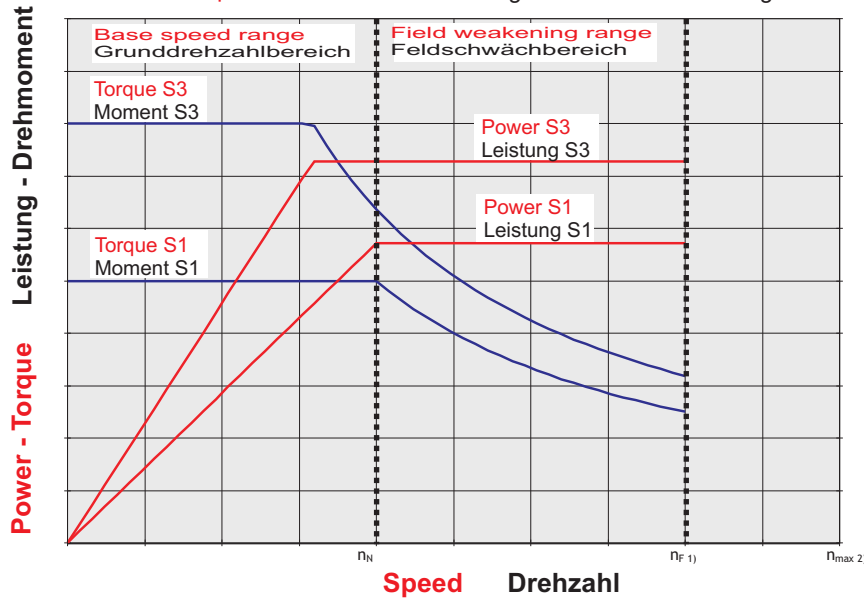
Power and torque characteristic Leistungs- und Drehmomentdiagramm
